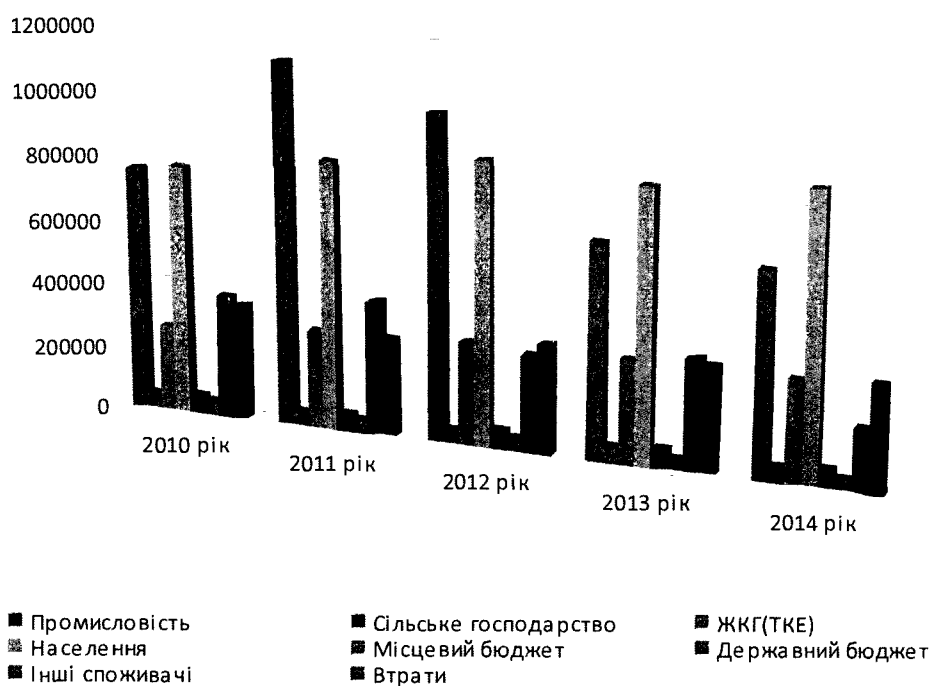
Діаграма 1.2.5. Споживання електричної енергії в розрізі груп споживачів Івано-Франківської області за період 2010-2014 роки, тис.кВт.год
